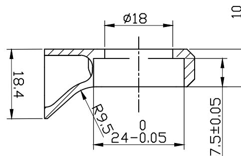
A-A Section
