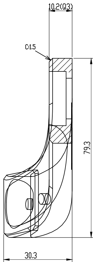
A-A SEC
