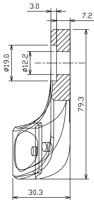
A-A SEC
