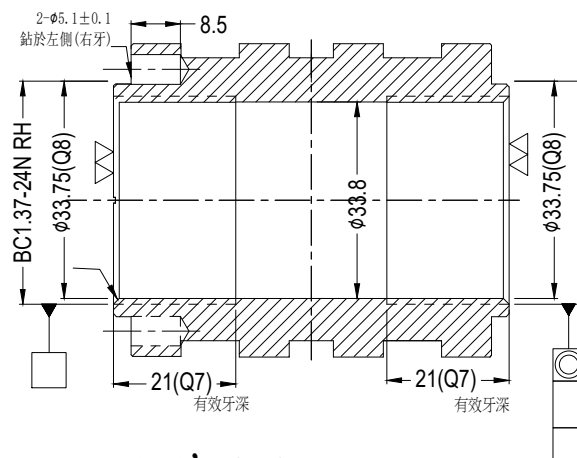
A-A' SEC
