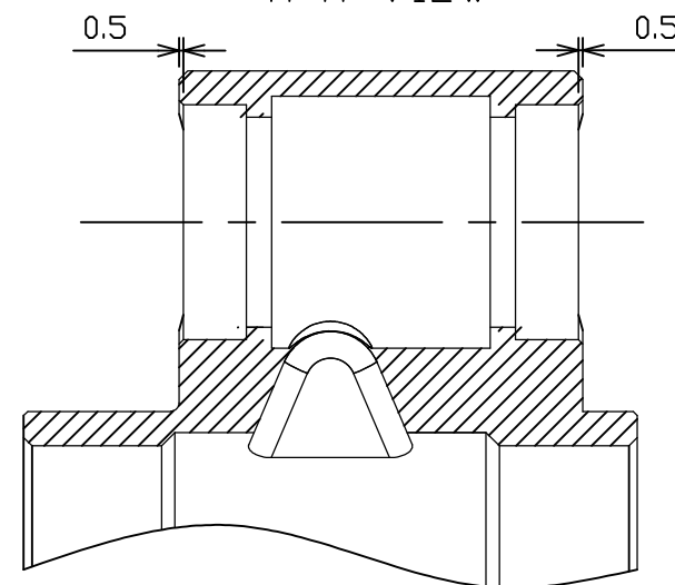
A-A VIEW
