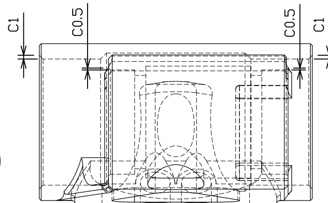
A-A VIEW
