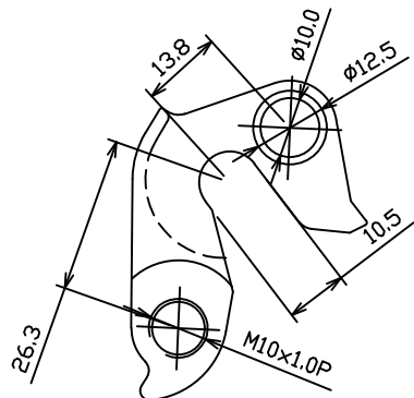
配 T-0022-1 吊耳
