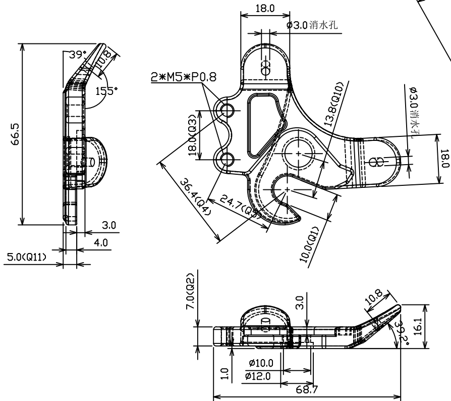
配 T-0022-1 吊耳
