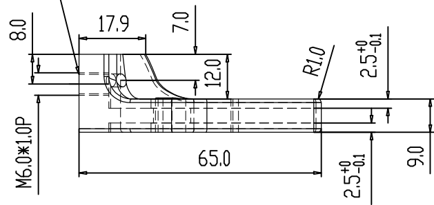
勾爪(左邊)(1PCS/SET)
